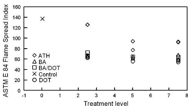
Fig. 7 Estimated ASTM E 84 flame spread index for samples Abb. 7 Geschätzter Flammenausbreitungsindex nach ASTM E 84
