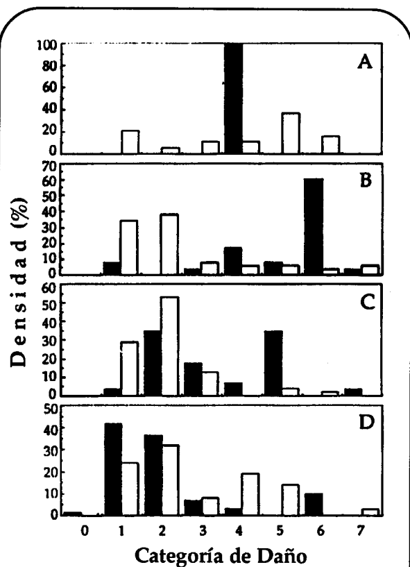
Figura 3. -Daño expresado como porcentaje de la densidad total de árboles para las especies Schefflera morototoni (A) y Miconia prasina (B), Tabebuia heterophylla (C) y Casearia arborea (D) en rodales de plantación (negro) y bosque secundario adyacente (blanco), Bosque Experimental de Luquillo. Daños según Tabla 1.
