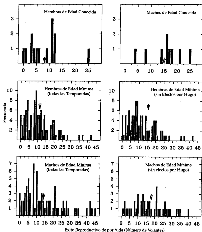
Figura 3. -Éxito reproductivo de por vida (expresado como número de volantones) en zorzales de edad conocida y mínima. El éxito reproductivo se comparó excluyendo los efectos del huracán Hugo mediante la eliminación de las temporadas de anidaje de 1990 y 1991. A pesar de que la distribución de frecuencias se ve alterada visualmente, no son significativas para cualquiera de los sexos a un nivel de confianza del 95%. Las flechas (↓) representan promedios.
