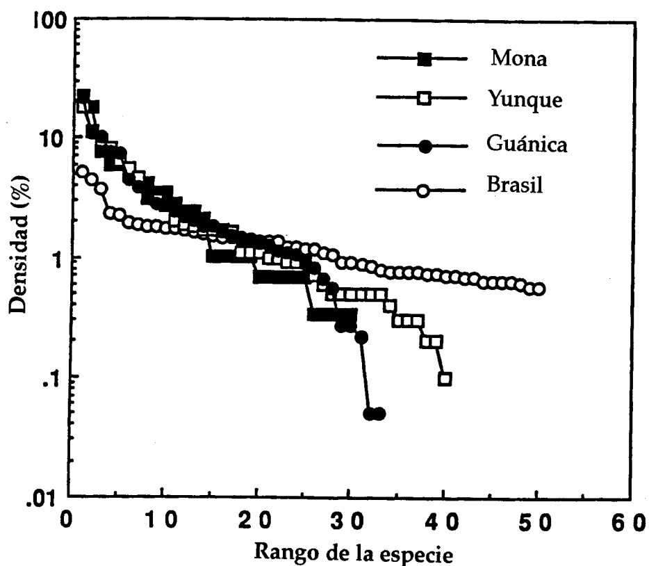
Figura 9. -Curvas de Importancia Relativa para la comunidad más diversa en la Isla de Mona (el bosque de la llanura), un bosque semidecidual maduro en Guánica, el bosque Experimental de Luquillo, y un bosque húmedo en la cuenca amazónica del Brasil (Lugo 1991).
