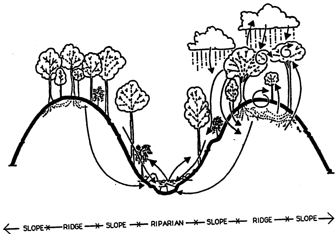
Figura 5. -Modelo de reciclaje de nutrientes en un bosque subtropical muy húmedo en Puerto Rico (Lugo y Scatena 1992). Las flechas ilustran los flujos de nutrientes y materia orgánica y definen las interfaces donde los organismos interactúan con el ambiente abiótico (tabla 4).
