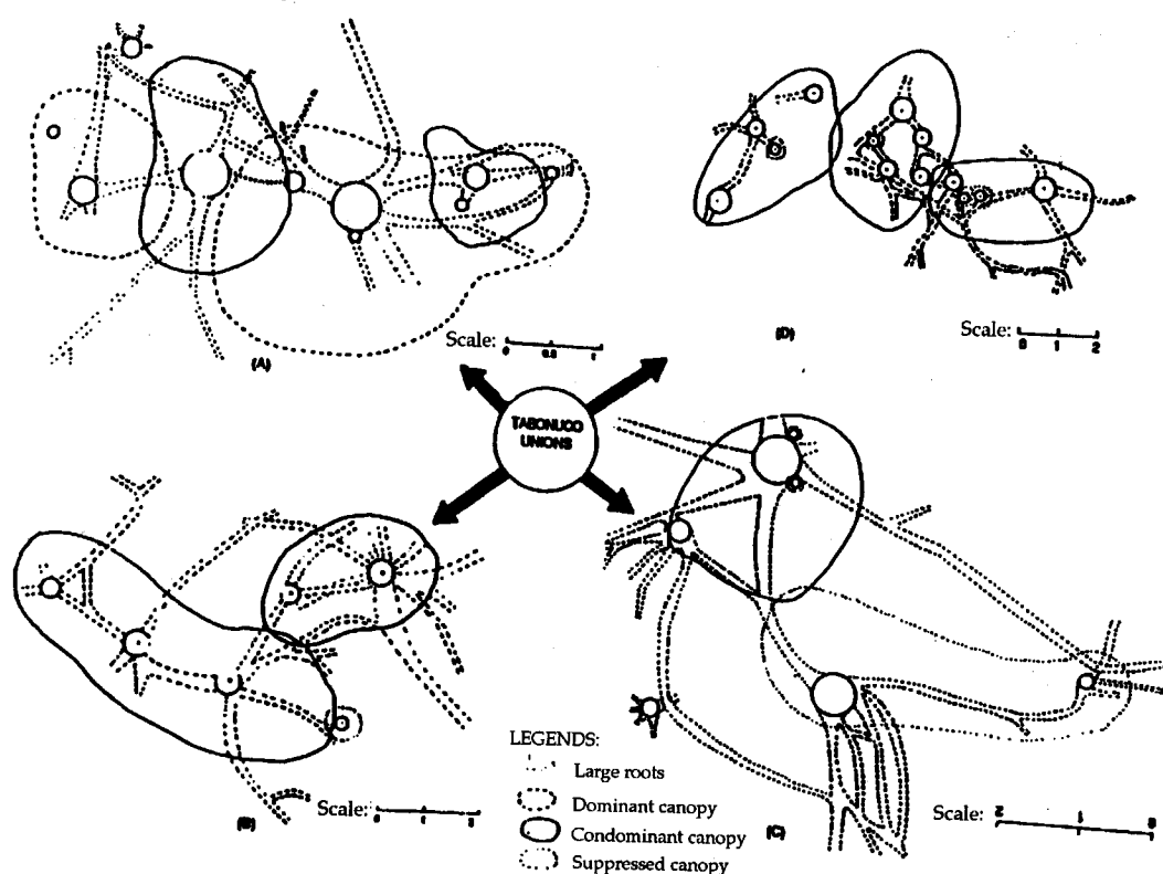
Figura 6. -Diagrama a escala de cuatro uniones de tabonuco en el Bosque de Luquillo (Basnet et al. 1993).
