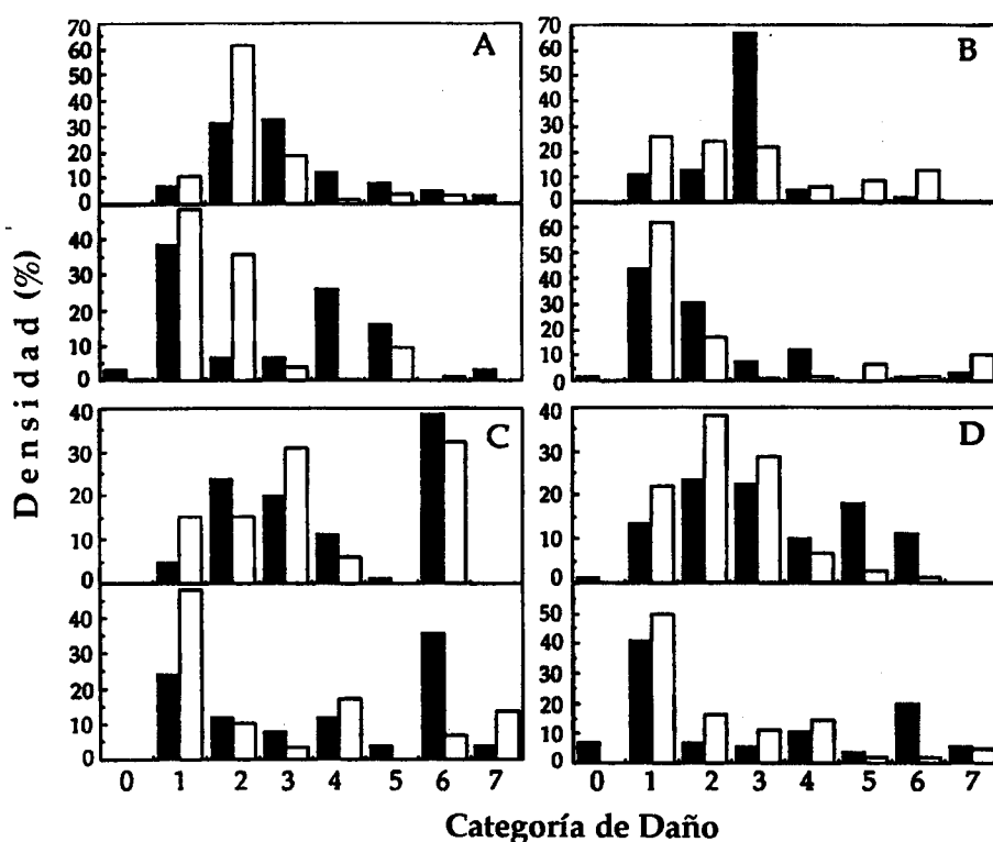
Figura 2. -Distribución de daños por clases de diámetro expresado como el porcentaje de la densidad total de árboles para los rodales de Guzmán (A), Cubuy (B), Sabana (C) y El Verde (D), en el Bosque Experimental de Luquillo. Las barras negras y blancas representan parcelas de plantación y bosque secundario respectivamente. Árboles con d.a.p. \geq 10 cm, gráfica superior y árboles con d.a.p. < 10 cm, gráfica inferior. Daños según Tabla 1.
