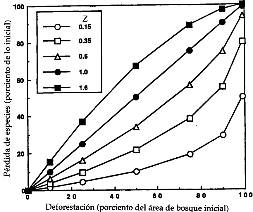
Figura 1. -Relación entre la deforestación y la pérdida de especies por extinción utilizando diferentes pendientes (factor Z) para la curva especie-área.
