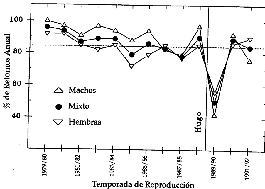
Figura 1. -Tasas de retorno anual para 86 machos y 121 hembras del Zorzal Pardo anidando en cajas entre 1979 y 1992. El huracán Hugo disminuyó las tasas de retorno de manera significativa, pero los niveles existentes previos al disturbio se recuperaron durante la segunda temporada de reproducción después del disturbio. La línea punteada que atraviesa todo el diagrama es la razón de retorno promedio para ambos sexos.
