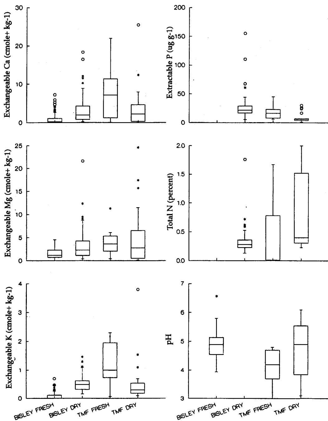
Figura 1. -Parcelas en forma de cuadrícula para el campo de valores de concentraciones de nutrientes en los suelos de superficie (0-10cm) de las Cuencas Hidrográficas de Investigación Bisley, el Bosque Experimental de Luquillo, Puerto Rico y otras ubicaciones de bosques tropicales montanos combinadas. Se comparan grupos de datos utilizando suelos frescos (Bisley Fresco, BTM Fresco) y suelos secos/de superficie (Bisley Seco, BTM Seco). Las barras representan la media entre los bigotes, las cuadrículas encierran el rango intercuartil, las estrellas representan los valores atípicos y los puntos son valores extremadamente atípicos (Silver et al. 1994).
