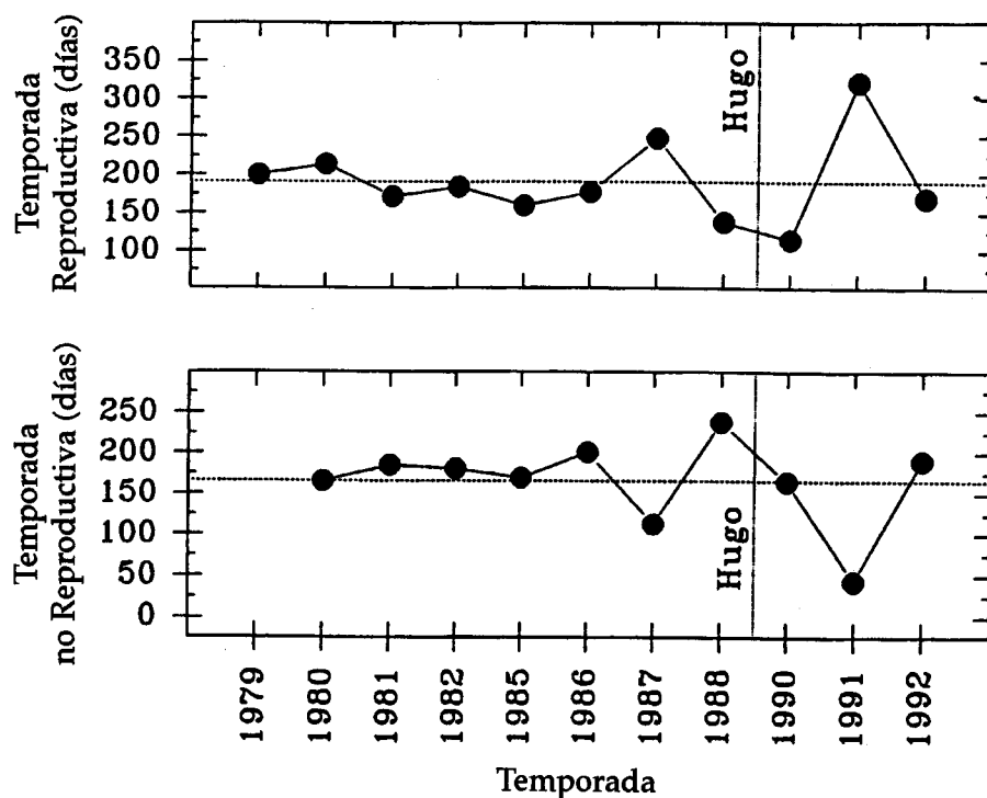
Figura 2. -Duración de las temporadas reproductivas y no-reproductivas para 11 Zorzales Pardos. Las líneas punteadas horizontales que atraviesan los diagramas representan la duración promedio de todas las temporadas reproductivas y no-reproductivas muestreadas entre 1979 y 1992. Los efectos del huracán Hugo sobre la duración de las temporadas reproductivas y no-reproductivas fueron significativos.
