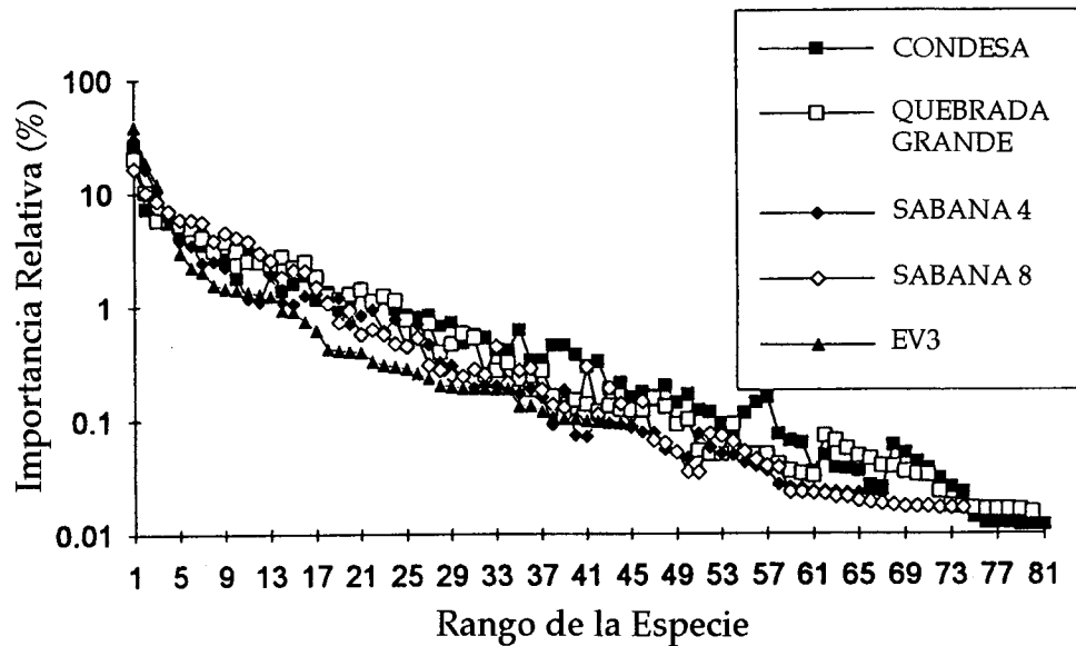
Figura 1. -Distribuciones lognormales (Whittaker 1965).
