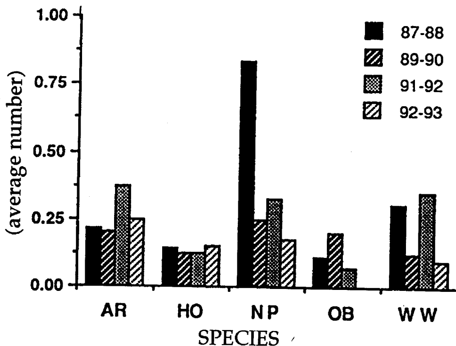
Figura 1. -Abundancia de cinco especies de reinitas residentes durante el invierno en St. John, Islas Vírgenes de los Estados Unidos. Número promedio de individuos por punto censado en el bosque húmedo (n=40) para las siguientes especies: ( Setophaga ruticilla (Sr), Mniotilta varia (Mv), Parula americana (Pa), Wilsonia citrina (Wc).
