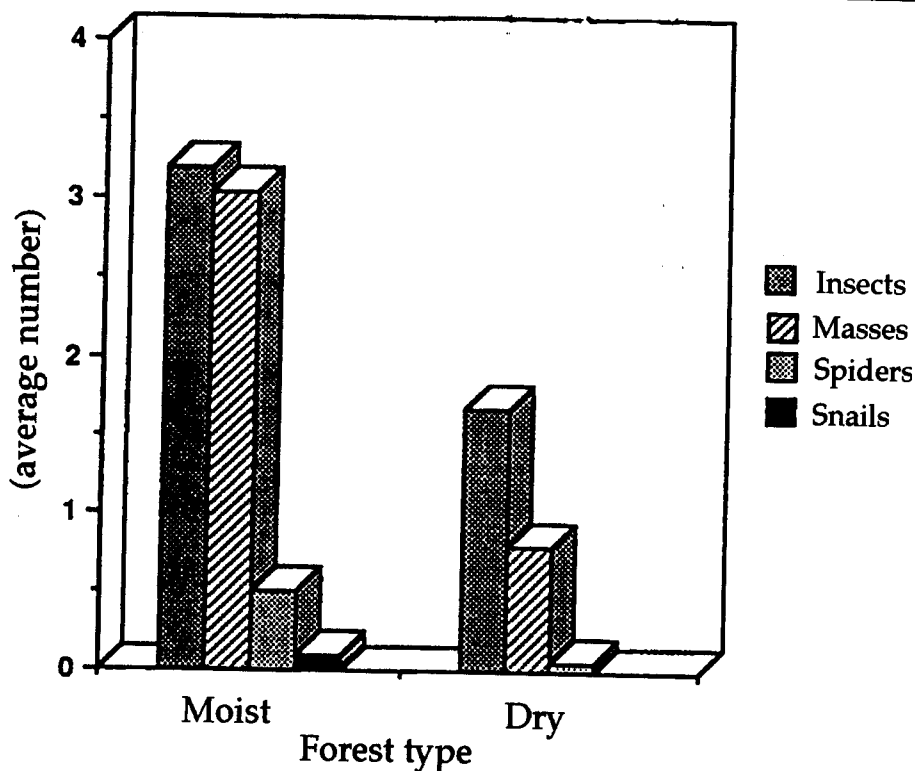
Figura 3. -Número de individuos promedio (para insectos, arañas y caracoles) o masas de individuos (agregaciones de huevos o insectos minúsculos como los áfidos). Se exponen los promedios para seis transectos en el bosque húmedo (moist) y tres transectos en arbolados secos (seco) que se censaron en un estudio preliminar.
