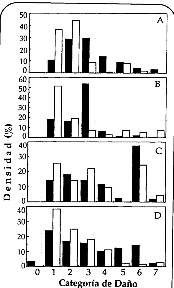
Figura 1. -Daño expresado como porcentaje de la densidad total de árboles para los rodales de Guzmán (A), Cubuy (B), Sabana (C) y El Verde (D) en el Bosque Experimental de Luquillo. Las barras negras y blancas representan parcelas de plantación y bosque secundario respectivamente. Daños según Tabla 1.
