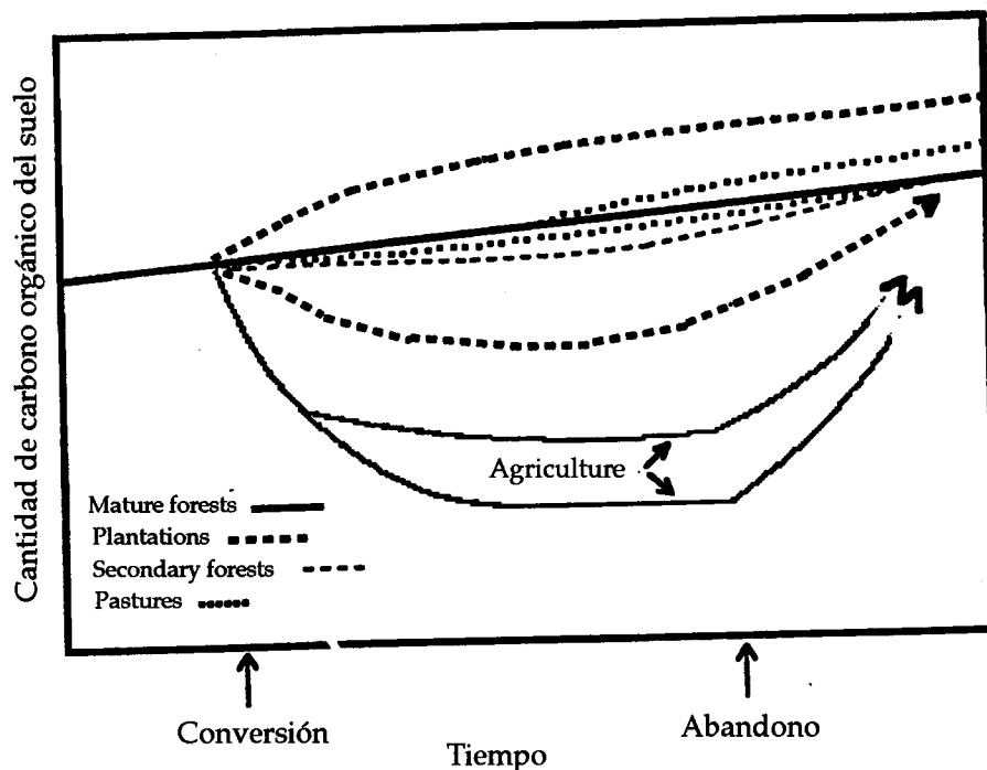
Figura 3. -Patrones sugeridos de cambio de carbono orgánico del suelo en suelo sujeto a diferentes usos de tierra en los trópicos. Este modelo ignora variaciones debido a tipo de suelo y conversiones mecánicas de localidades. El tipo de uso agrícola o especies de plantaciones sembradas cambia la pendiente de las curvas (Lugo y Brown 1992).
