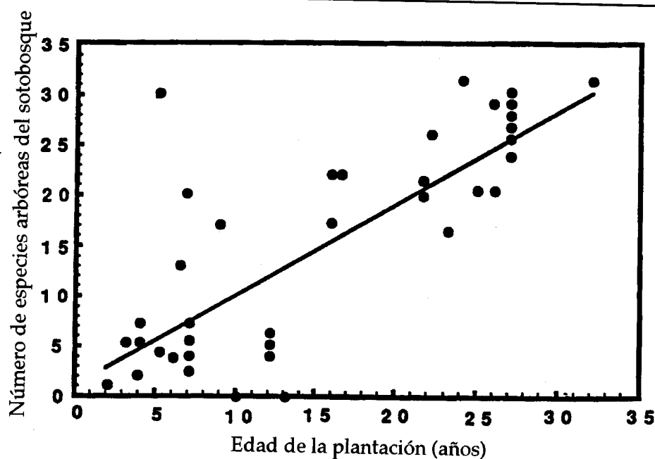
Figura 2. -Relación entre el número de especies de árboles en el sotobosque de plantaciones de árboles y la edad de la plantación (Lugo et al. 1993). La relación para estos datos es y=0.74+ 0.93 x , ( r^2 = 0.62 ).
