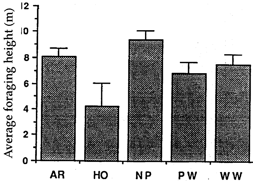
Figura 2. -Alturas de forrajeo promedio para las cinco especies de reinitas observadas con mayor frecuencia en un estudio preliminar. El tamaño de las muestras son como sigue: Las barras representan el error estándar.
