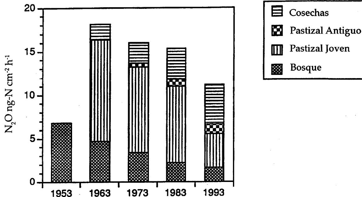
Figura 2. -Emisiones del ( N_2O ng-N cm^{-2} h^{-1} ) estimado para Sarapiquí desde 1953 hasta 1993.
