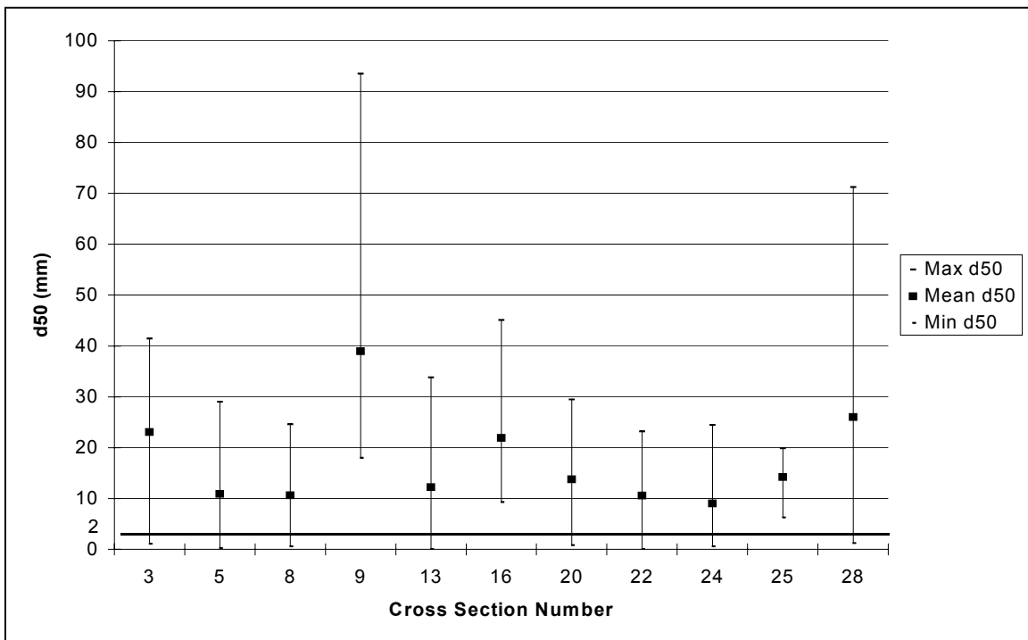
Fig. 3.21. 1995 median bed material size data.
