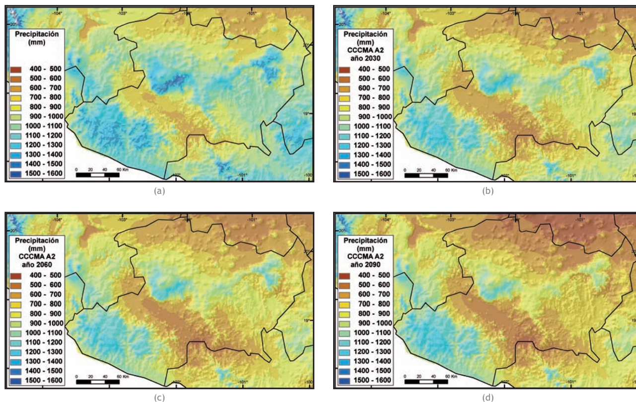
Figura 6. Mapa de Michoacán de predicciones de precipitación anual (mm de lluvia) para: (a) clima contemporáneo (promedio 1960-1990), (b) año 2030, (c) año 2060, y (d) año 2090. Predicciones basadas en datos del Centro Canadiense para el Modelaje y Análisis del Clima (CCCMA), escenario de emisiones A2. Fuente: Basado en Sáenz-Romero et al. 2009.
