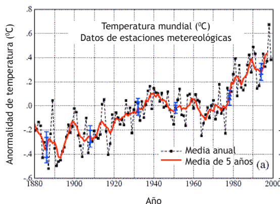
Incremento de temperatura (1880 - 2000). Fuente: Basado en Weart 2008.
