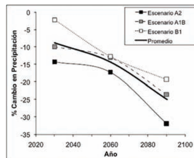
Figura 3. Decremento estimado de la precipitación total anual, expresado como porcentaje de cambio respecto a la precipitación contemporánea; promedio para Michoacán para los años 2030, 2060 y 2090. Estimaciones a partir del modelo canadiense, para tres escenarios de emisiones (B1 “optimista”, A1B “intermedio” y A2 “pesimista”), y promedio entre los tres escenarios (línea gruesa).
