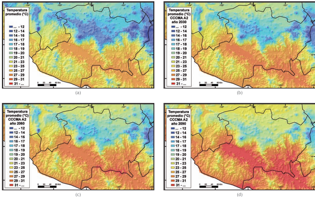
Figura 5. Mapa de Michoacán de predicciones de temperatura media anual (°C) para: (a) clima contemporáneo (promedio 1960-1990), (b) año 2030, (c) año 2060, y (d) año 2090. Predicciones basadas en datos del Centro Canadiense para el Modelaje y Análisis del Clima (CCCMA), escenario de emisiones A2. Fuente: Basado en Sáenz-Romero et al. 2009.
