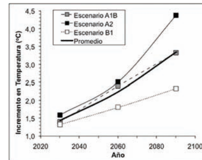
Figura 2. Incremento estimado de temperatura anual promedio para Michoacán para los años 2030, 2060 y 2090, en comparación al clima contemporáneo. Estimaciones a partir del modelo canadiense, para tres escenarios de emisiones (B1 “optimista”, A1B “intermedio” y A2 “pesimista”), y promedio entre los tres escenarios (línea gruesa).
