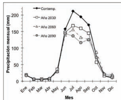
Figura 4. Precipitación promedio mensual, contemporánea y para los años 2030, 2060 y 2090, promedio para Michoacán. Estimaciones a partir del modelo canadiense, escenario de emisiones A2.
