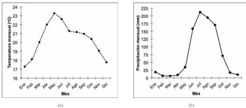
Figura 1. Clima contemporáneo promedio de Michoacán, basado en datos de 30 años (1960-1990) de 149 estaciones climáticas. (a) Promedio mensual de temperatura (grados centígrados, °C), y (b) Promedio mensual de precipitación (milímetros de lluvia, mm).
