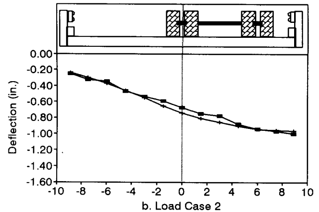
b. Load Case 2
