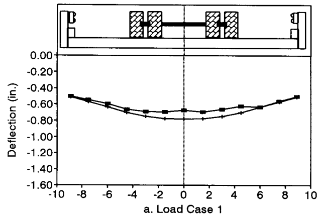
a. Load Case 1
