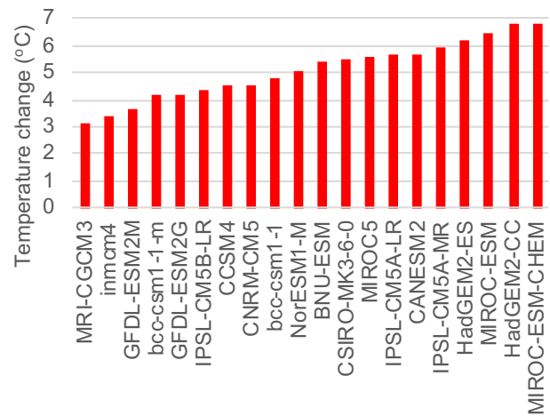
(d) RCP 8.5
