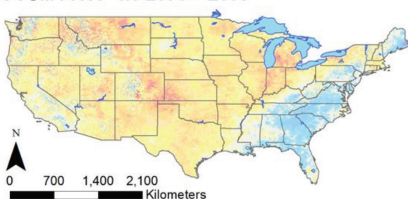
CCSM4 RCP 4.5 2070 – 2099
