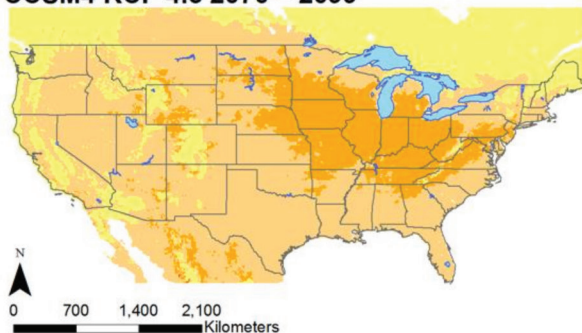
CCSM4 RCP 4.5 2070 – 2099
