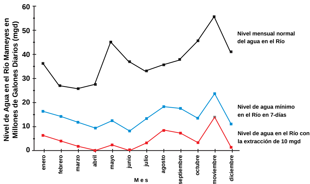
Figura 2 —Efectos sobre el nivel del agua del Río Mameyes de la extracción de 10 mgd propuesta por la AAA (Programa I).
